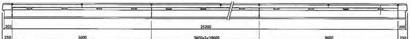
コースロープ収納ベンチ本体図
