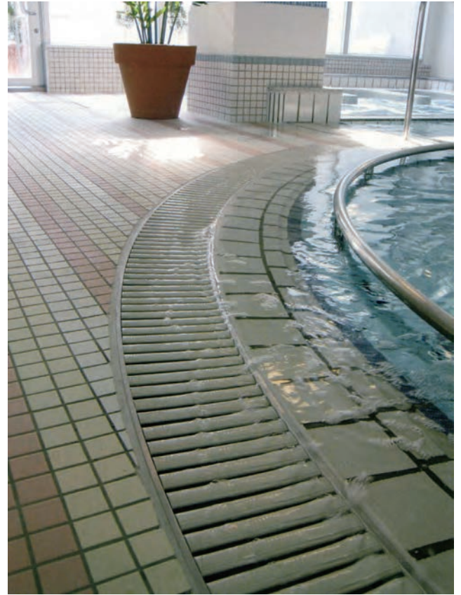
比重が重いため、浮きにくい構造です。(比重1.2)
