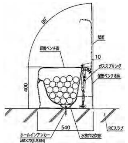
コースロープ収納ベンチ断面図
